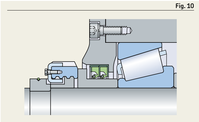
HDSE1 seal
