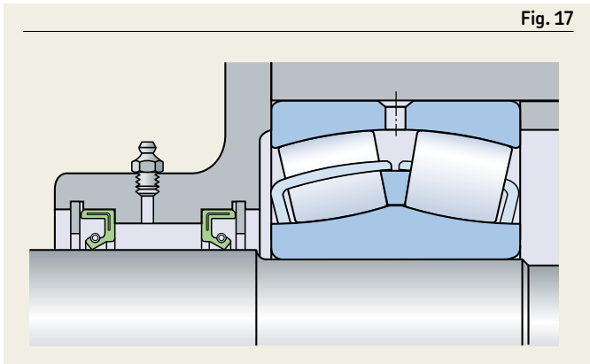
HMS5 seals
